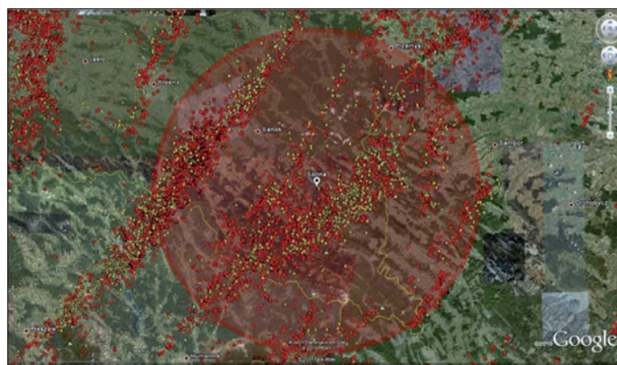
Fot. 2. Graficzna reprezentacja przykładowych danych systemu LINET dla rejonu Bieszczad z 19 lipca 2011 r. (znaczniki czerwone – wyładowania doziemne, znaczniki żółte – wyładowania w chmurach)
