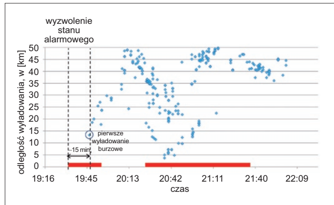
Rys. 2. Porównanie wskazań systemu Thor Guard z danymi systemu LINET z 8 sierpnia 2011 r.
