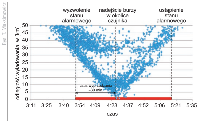
Rys. 1. Porównanie wskazań systemu Thor Guard z danymi systemu LINET z 19 lipca 2011 r.
