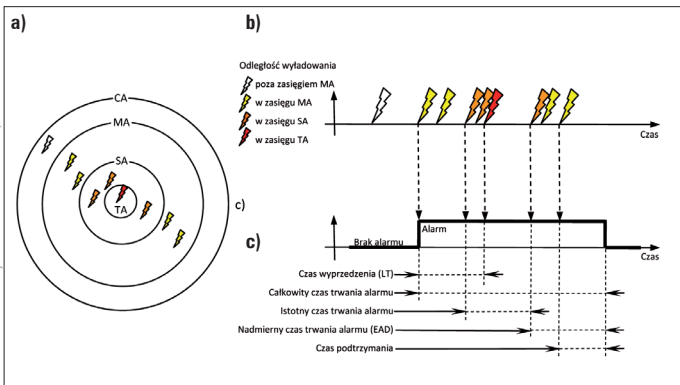
Rys. 1. Przykład wyzwalania alarmu: a) lokalizacja wyładowań w zdefiniowanych obszarach, b) czas wystąpienia wyładowań, c) czas wyzwolenia alarmu
